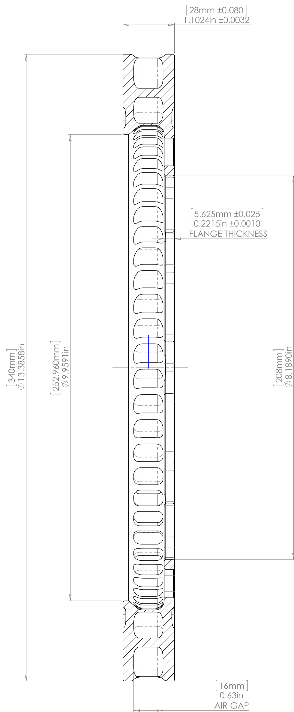
SECTION A-A
